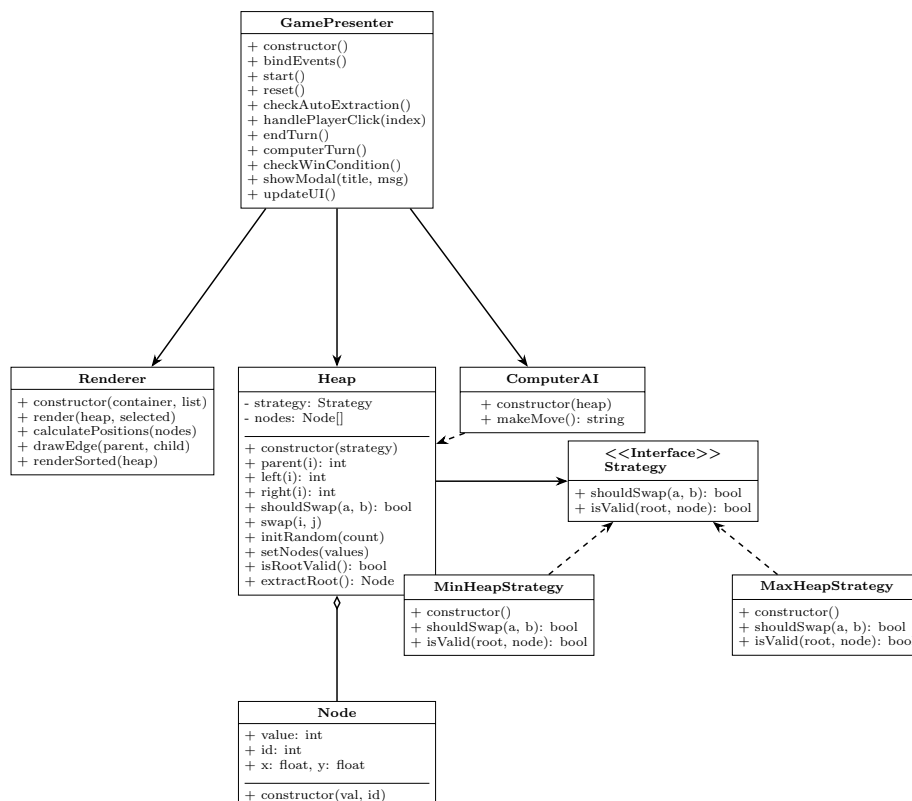
Figura 3.8: Diagramma delle Classi - Architettura MVP
